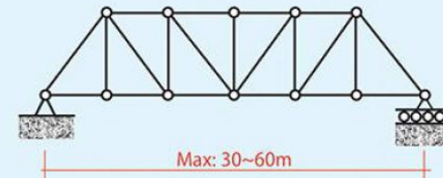
PRATT
