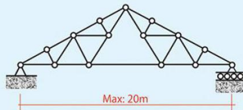
FINK
